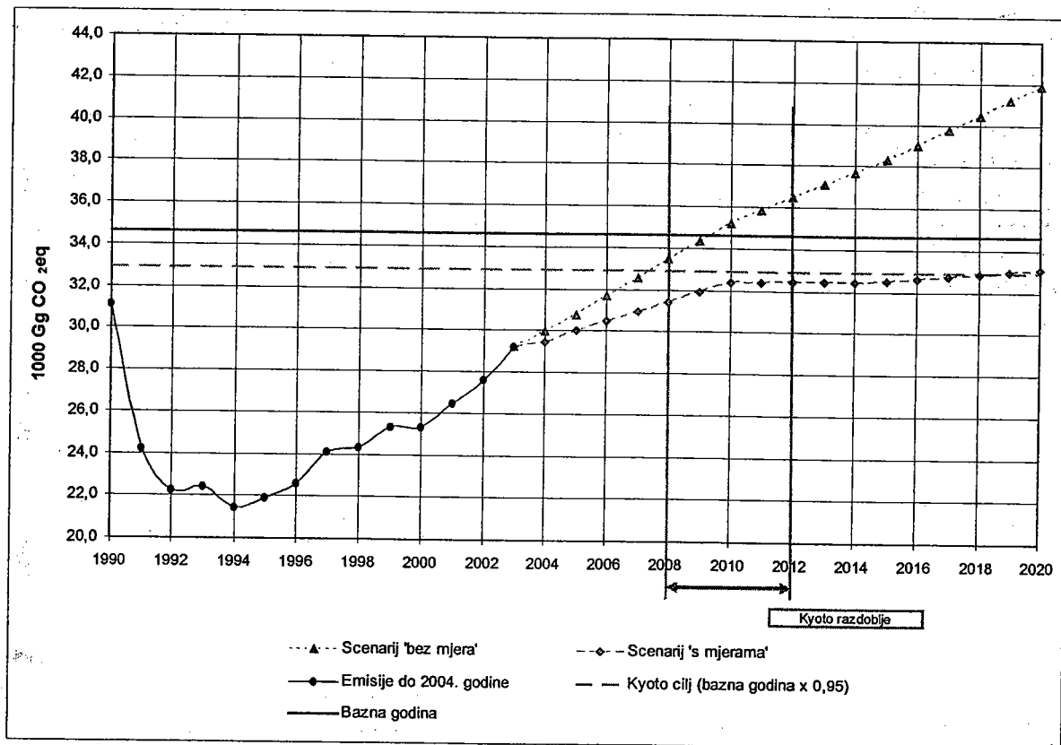
Slika 1: Projekcije emisije stakleničkih plinova u Republici Hrvatskoj do 2020. godine
